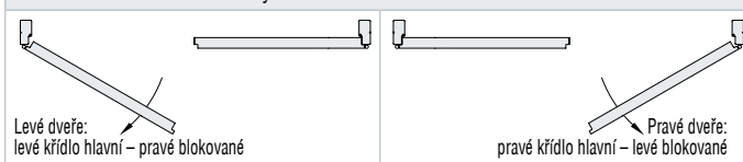
Směry otevírání – dvoukřídlé dveře falcové
