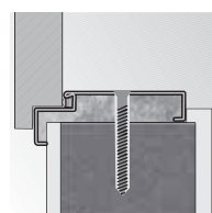
rohová zárubňa veľká montáž pomocou príchytiek
