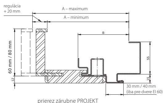
prierez zárubne PROJEKT
